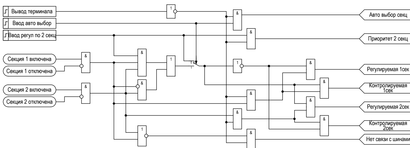
Рисунок 2.7 – Функциональная схема логики выбора регулируемой секции
